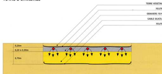
COUPE TRANSVERSALE
